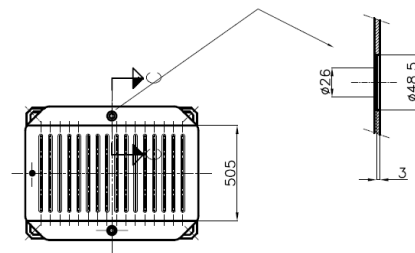
CORTE C-C E.:6/1
