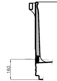
SECCION POR A-A E.:2/1
