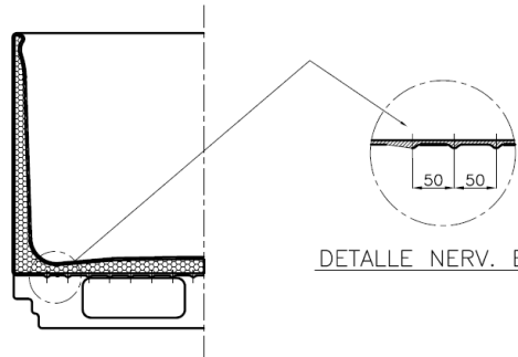
SECCION POR B-B E.:2/1
