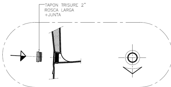
DETALLE SALIDA ROSCADA E.:3/1
